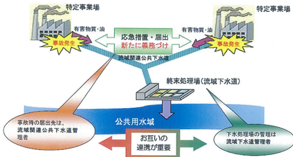
図-3.4 流域下水道における連携の重要性
